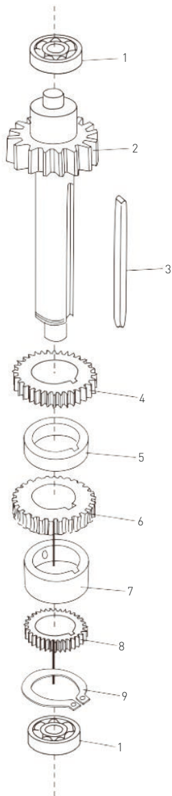
Abb. 3: Baugruppe der Getriebeachse
