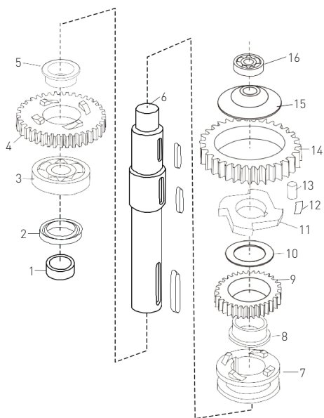
Fig. 2: Unità dell'asse
