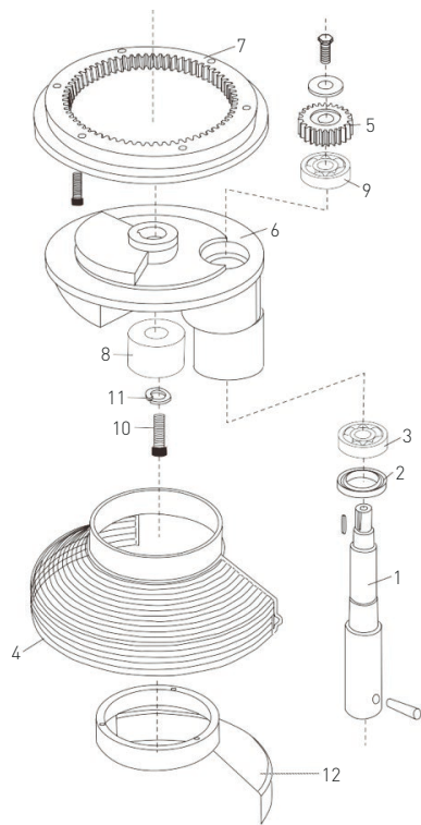
Figura 6: Placa rotativă și axul de malaxare
