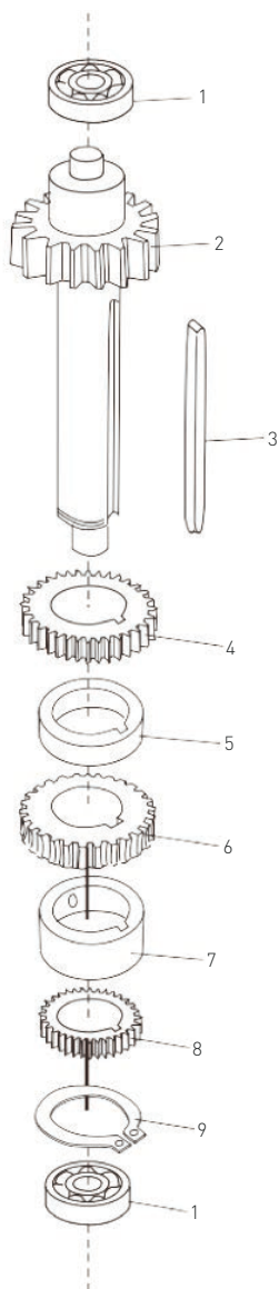
Εικόνα 3: Διάταξη άξονα γραναζιών
