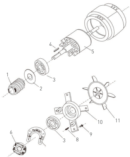
Rys. 4: Zespół silnika
