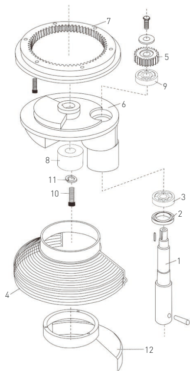
Fig. 6 : Plaque rotative et l'axe de mélange
