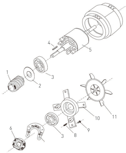
Abb. 4: Motorbaugruppe
