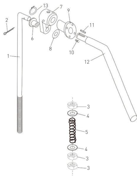
Rys. 5: Zespół podnośnika misy
