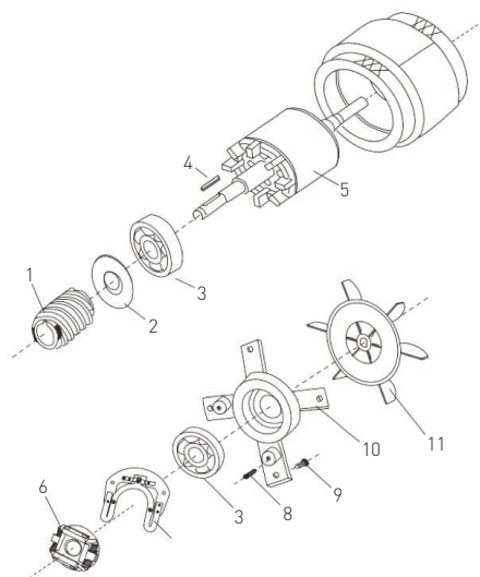
Εικόνα 4: Διάταξη μοτέρ
