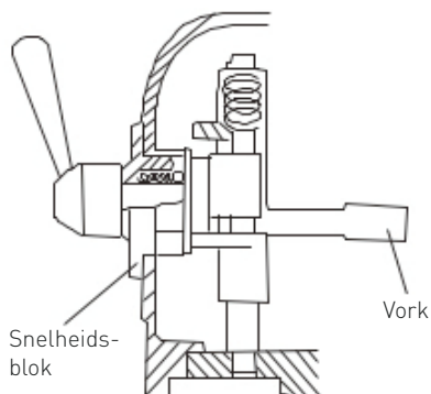
Figuur 7: Snelheidsregeling
