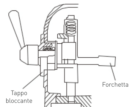
Fig. 7: Unità di impostazione della velocità
