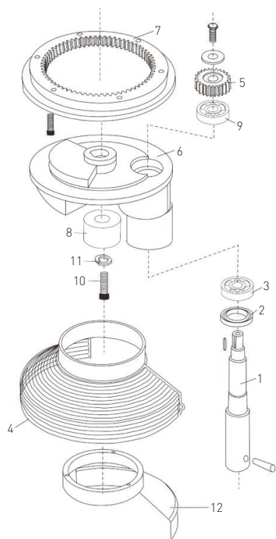
Рис. 6: Вращательная пластина и смесительная ось
