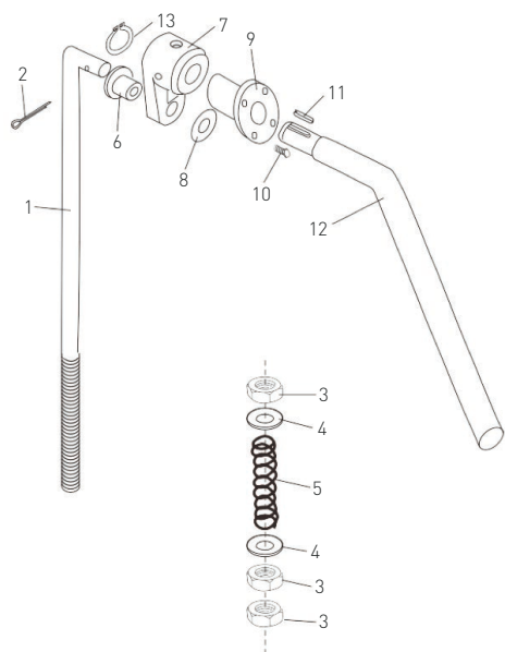
Рис. 5: Узел подъема чаши
