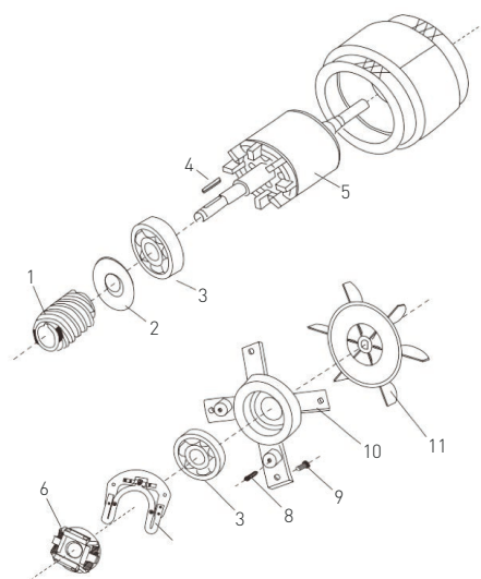
Figura 4: Ansamblu motor
