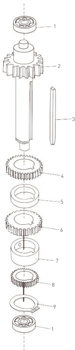
Figuur 3: Tandwielas
