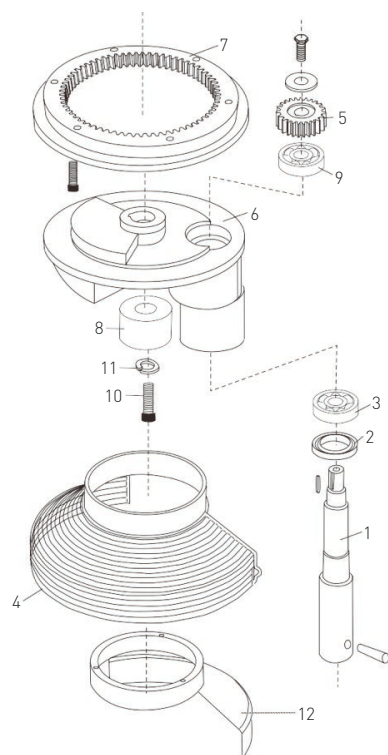
Rys. 6: Płyta obrotowa i oś mieszająca
