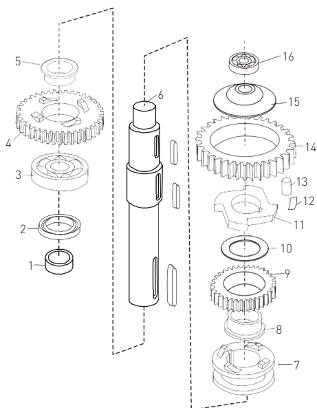
Рис. 2: Узел оси
