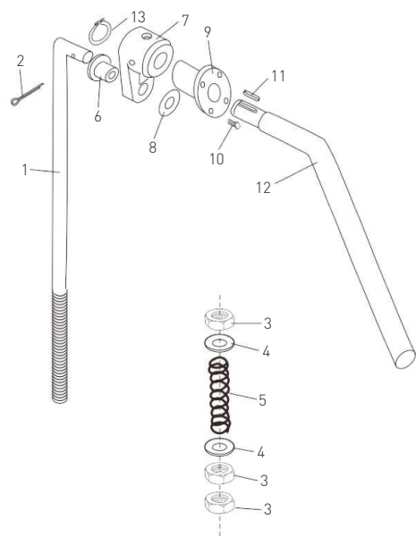
Figuur 5: Mechanisme heffen kom
