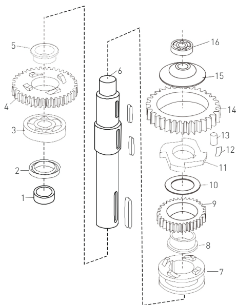
Εικόνα 2: Διάταξη άξονα
