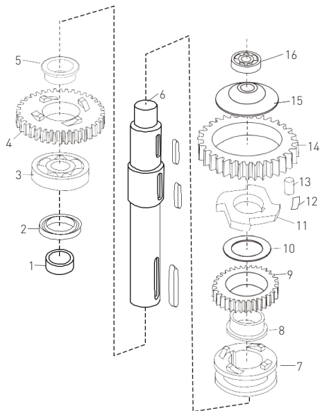
Rys. 2: Zespół osiowy
