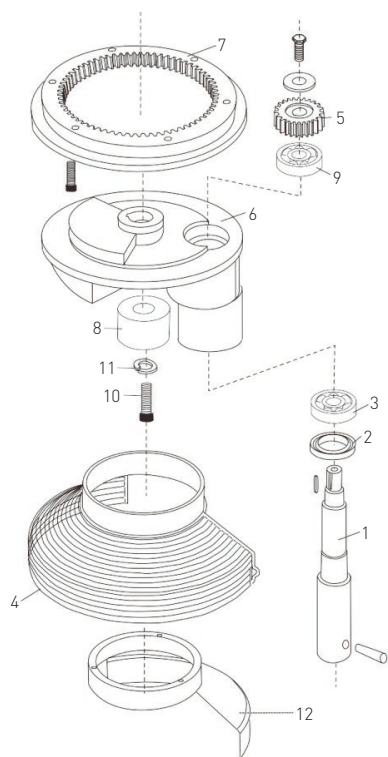
Abb. 6: Drehplatte und Mischachse
