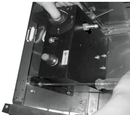
ΒΗΜΑ 2: Φροντίστε η δεξαμενή να κοιτάζει προς τα κάτω. Στερεώστε τον καυστήρα (J) στη δεξαμενή χρησιμοποιώντας τις 4 κλασσικές βίδες και τις ροδέλες (BB).
