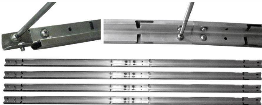
ΒΗΜΑ 3: Αφαιρέστε τις 2 βίδες και τις ροδέλες (BB) από τη μπάρα στήριξης - κάτω (F). Εισάγετε τη μπάρα στήριξης - άνω (E) στη μπάρα στήριξης - κάτω (F) και στερεώστε τη χρησιμοποιώντας τις 2 κλασσικές βίδες και ροδέλες (BB). Επαναλάβετε αυτό το βήμα για να συνδέσετε τις 3 αριστερές μπάρες στήριξης.
